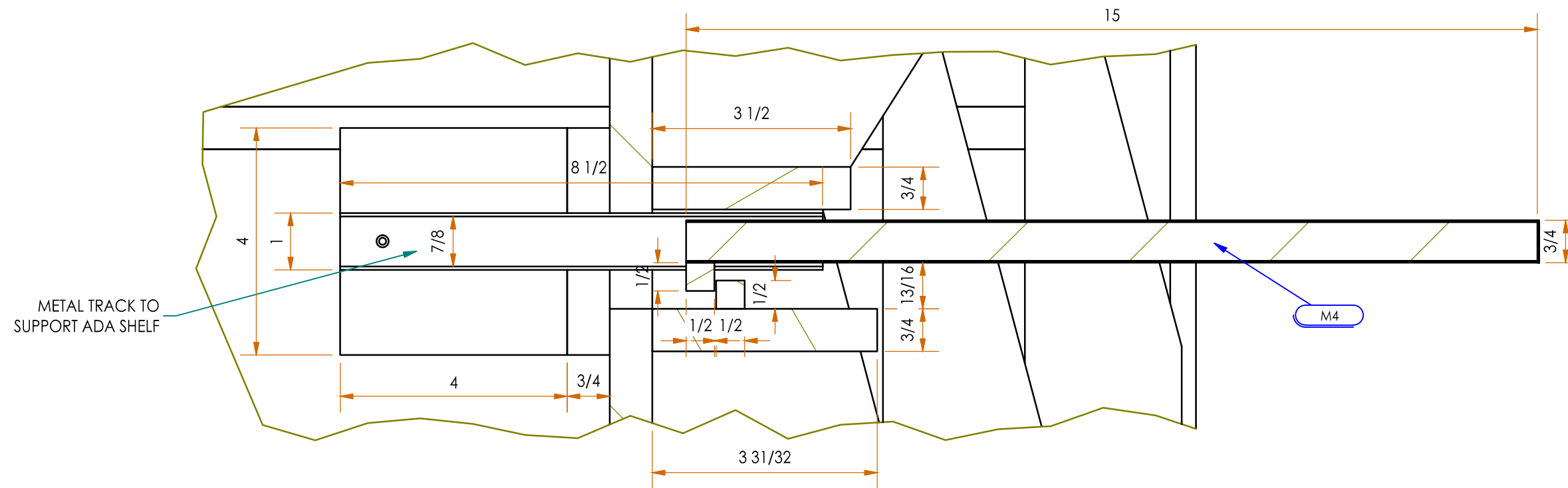
ADA SHELF DETAIL
