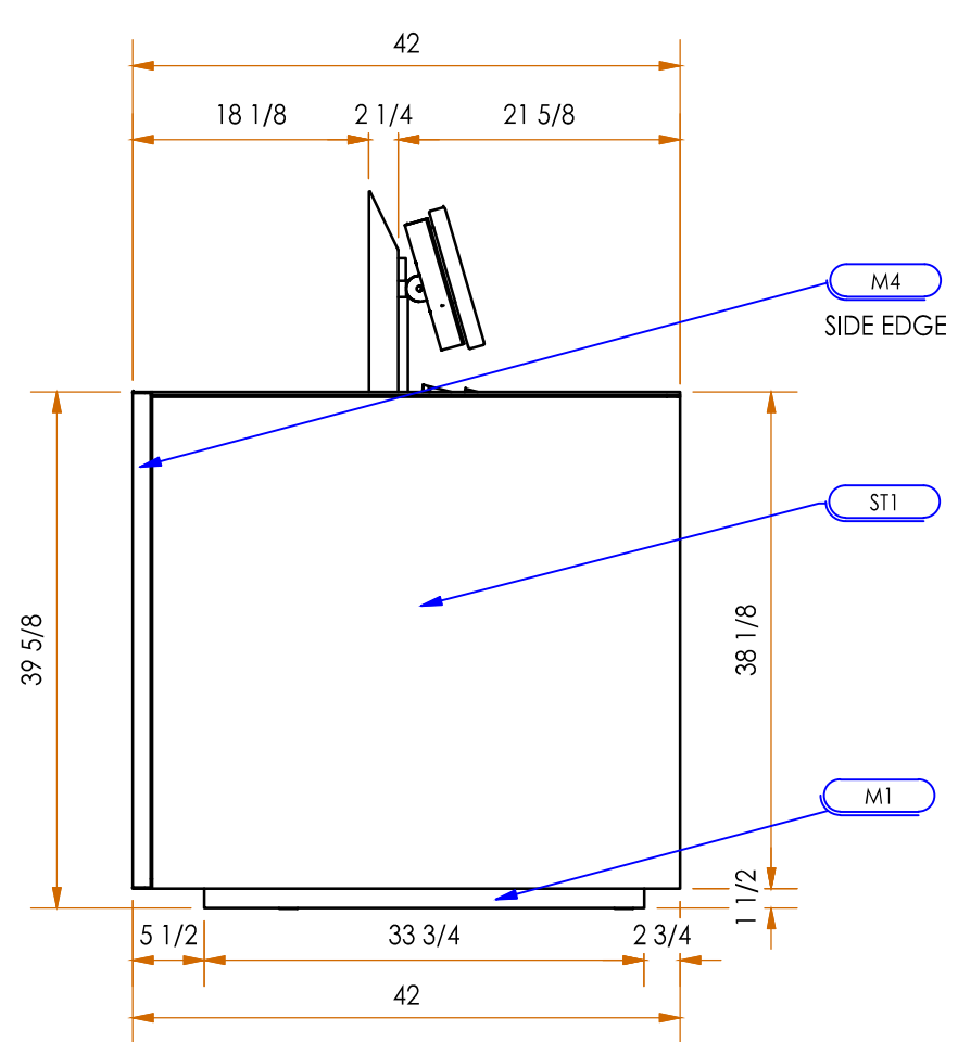
RIGHT ELEVATION
